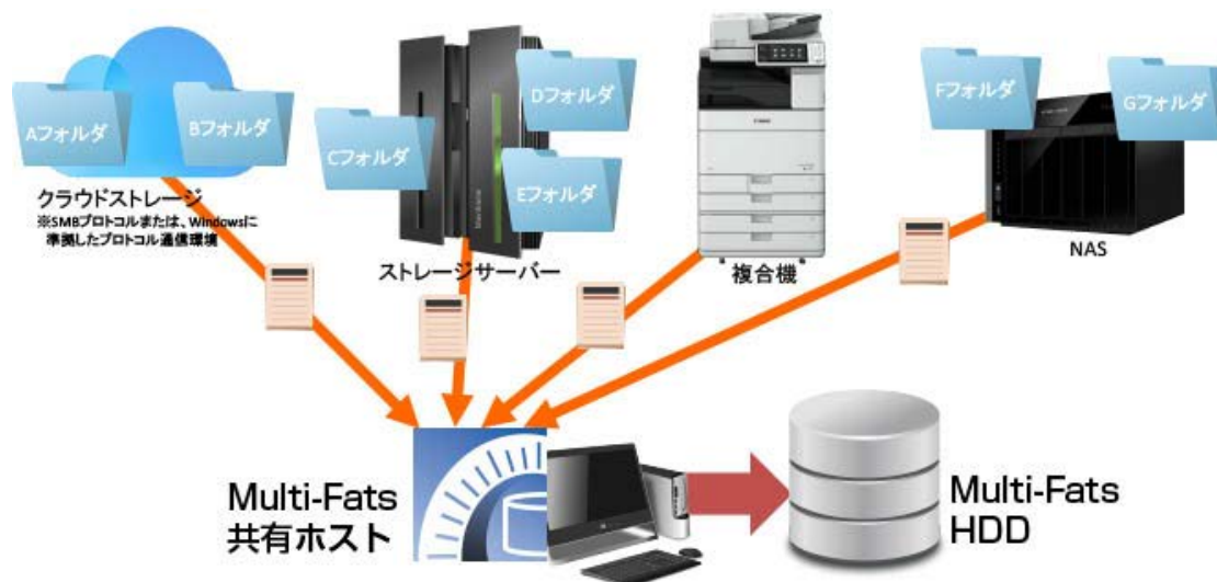
Share 版システム構成
